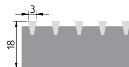
Разрез профиля
