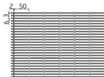
Вид сверху
